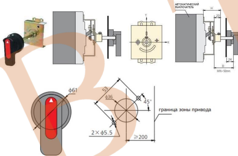
Установочные размеры ручного привода управления.
