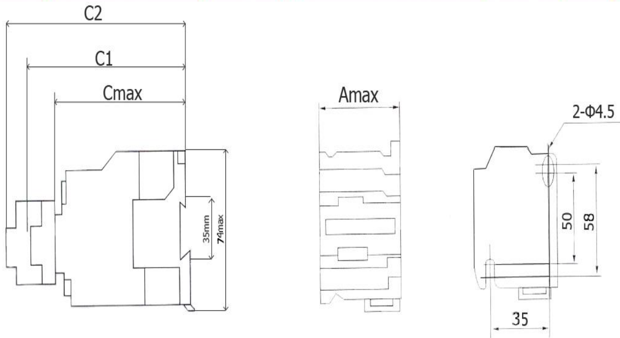
Рисунок 1 – Габаритные и присоединительные размеры пускателей 9-12А
